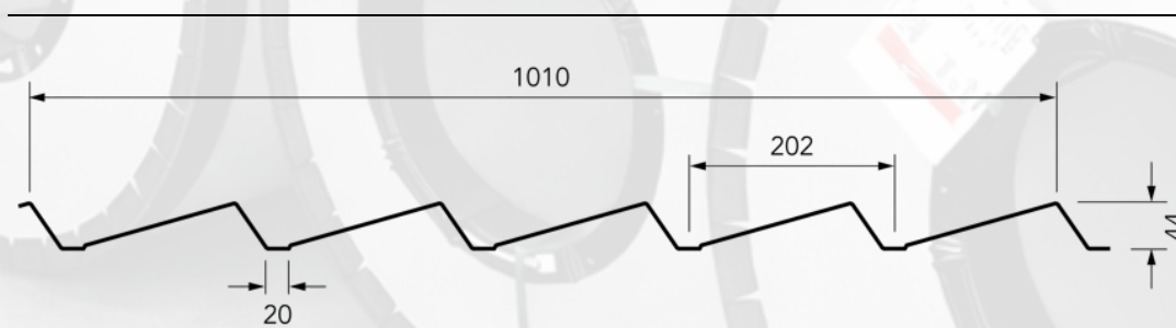
DETALLE SECCIÓN CHAPA
