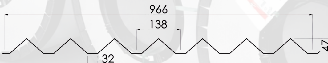
DETALLE SECCIÓN CHAPA
